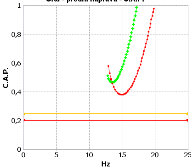
Graf - přední náprava - C.A.P.
